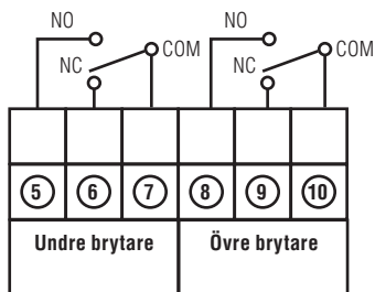
Inkoppling av mekaniska- och proximitybrytare
