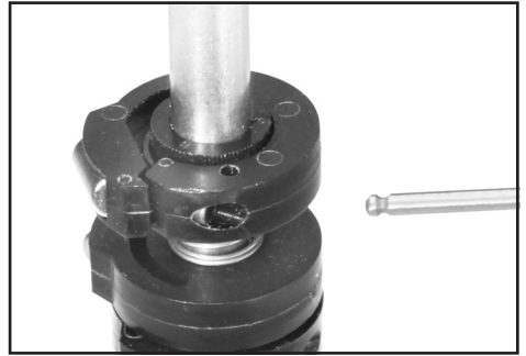
微调凸轮
